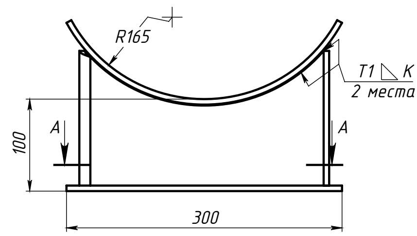
Поз.3 (Ложемент)
