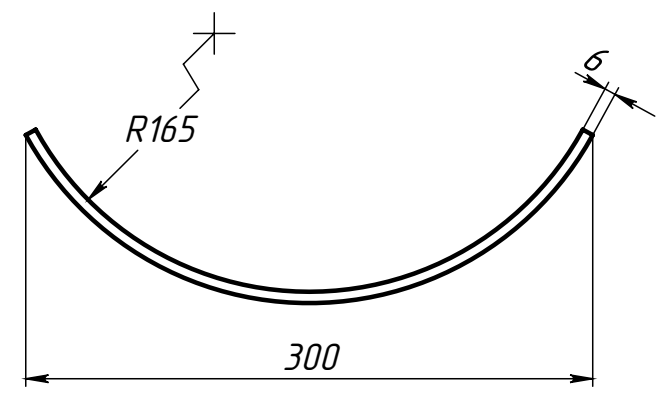
Поз.3 (Ложемент)
